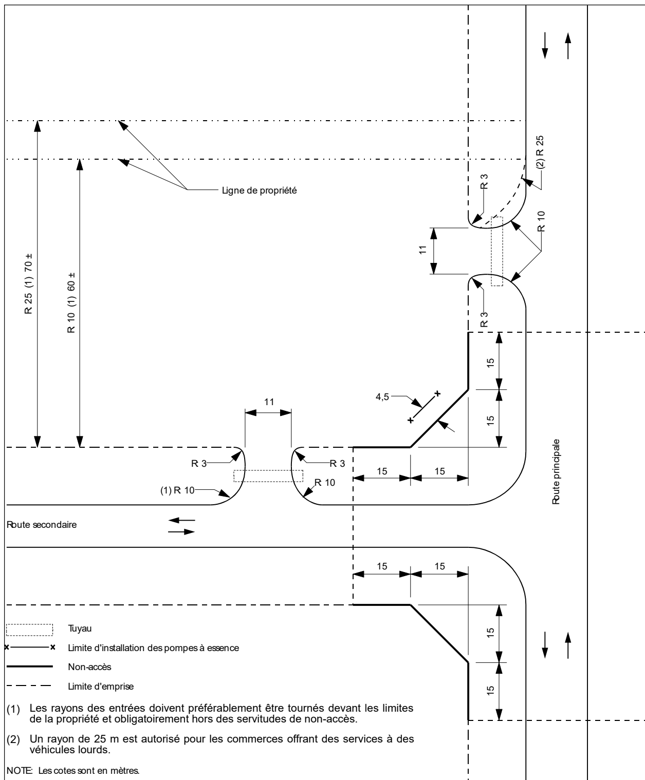
FIGURE 4.14.6.4a : ENTRÉE COMMERCIALE À UNE INTERSECTION
