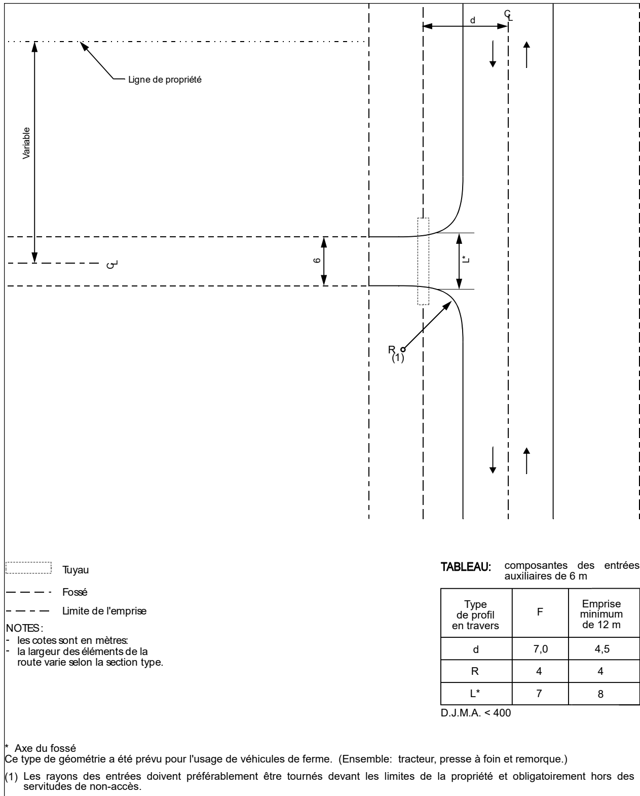
FIGURE 4.14.8.4 : ENTRÉE DE CHAMP
