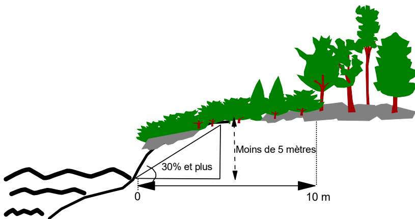
Figure 4.5.1b : Rive de 10 mètres (cas no.2)
