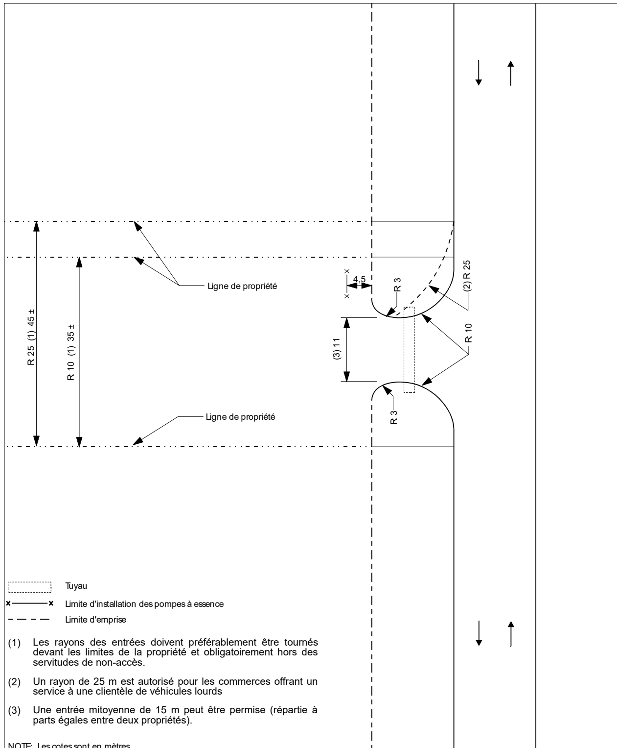
FIGURE 4.14.6.4c : ENTRÉE SIMPLE COMMERCIALE HORS INTERSECTION
