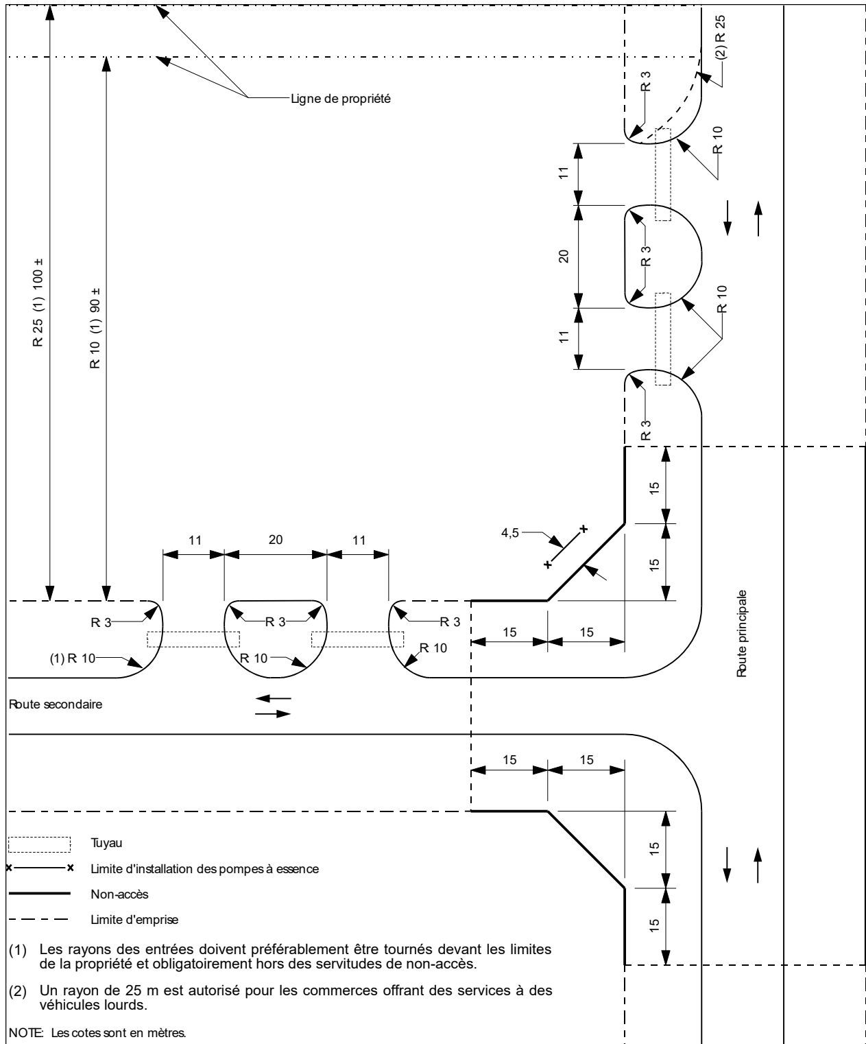
FIGURE 4.14.6.4b : ENTRÉE COMMERCIALE À UNE INTERSECTION
