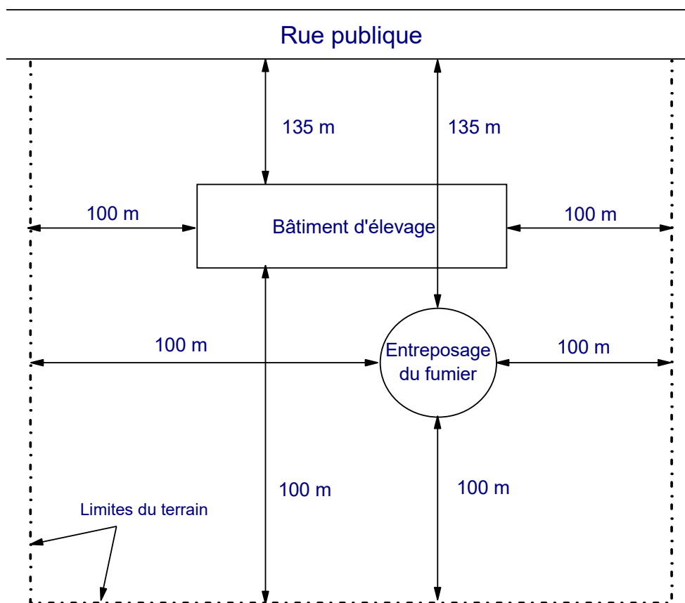
FIGURE 4.15.4.1 : MARGES DE REcul
