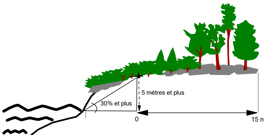
Figure 4.5.1d : Rive de 15 mètres (cas no.2)
