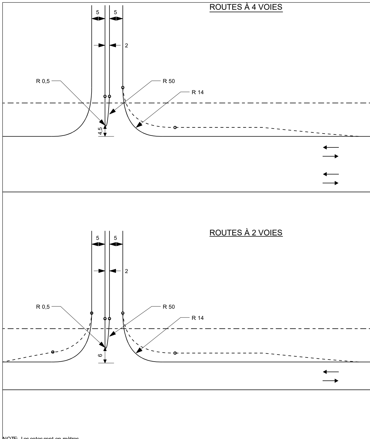
FIGURE 4.14.6.4e : ENTRÉE COMMERCIALE À GRANDES SURFACES (UNE ENTRÉE ET UNE SORTIE)
