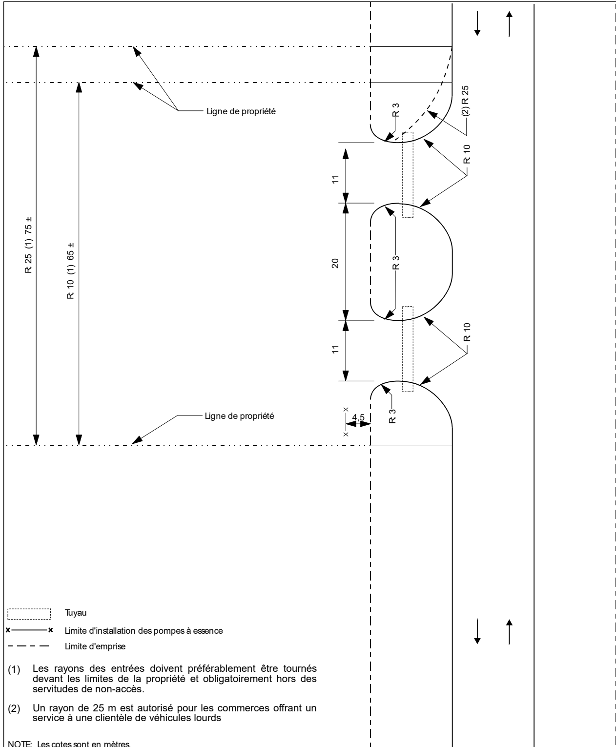
FIGURE 4.14.6.4d : ENTRÉE COMMERCIALE HORS INTERSECTION (2 ENTRÉES)
