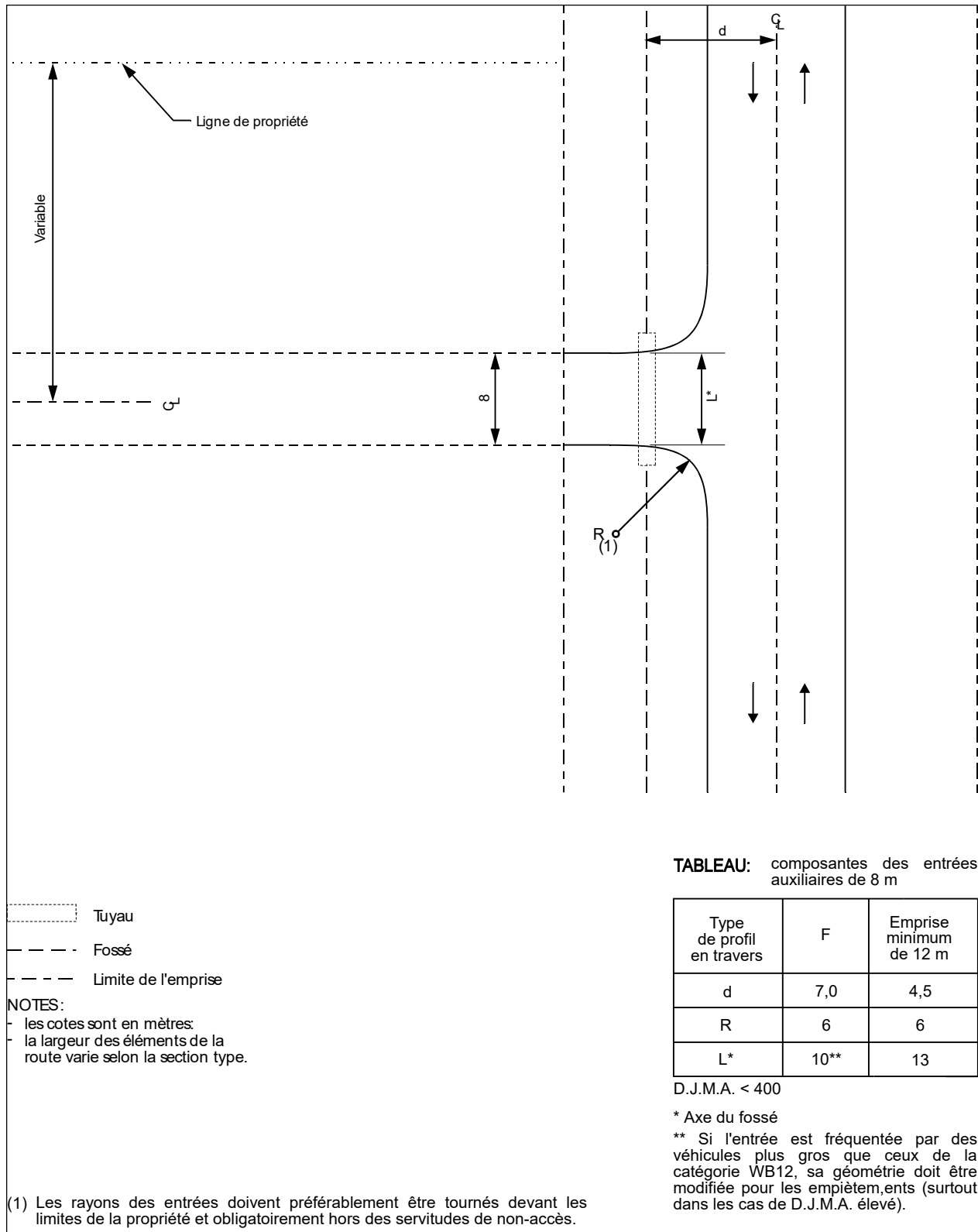
FIGURE 4.14.7.4 : ENTRÉE PRINCIPALE DE FERME
