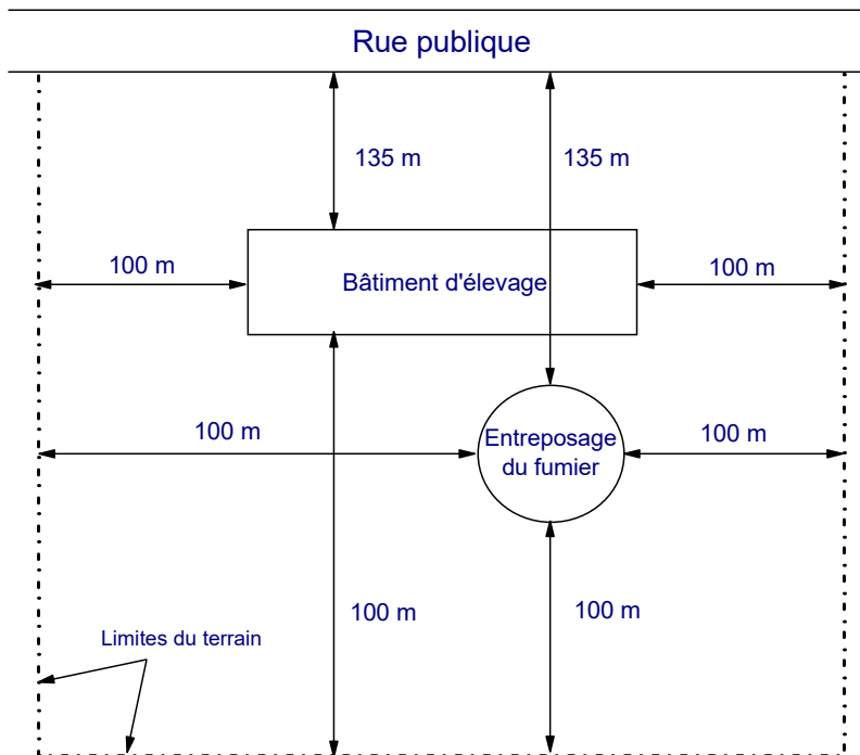
FIGURE 21.6 : MARGES DE REcul
